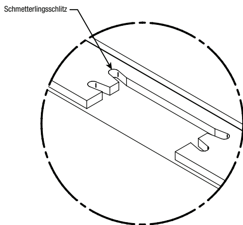
ABBILDUNG 14: SPANNFEDEREINRASTSCHLITZ
