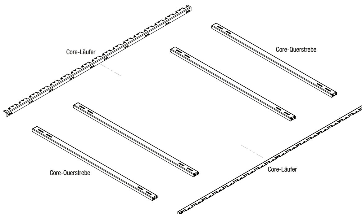
ABBILDUNG 3: CORE QUERSTREBEN
