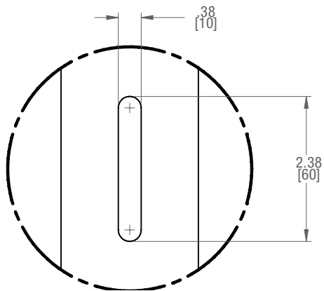
ABBILDUNG 4: CORE SCHLITZABMESSUNG
