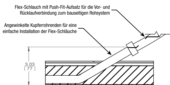
ABBILDUNG 20: SCHLAUCHINSTALLATION
